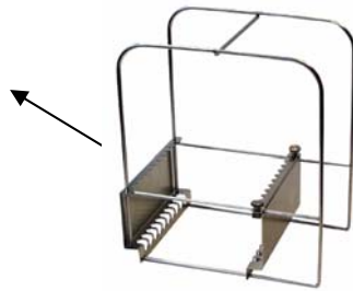
Plattenhalter LP 14 - verstellbar für unterschiedliche Größen (Einhängekorb erforderlich)
